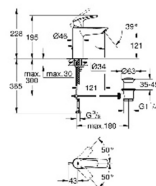
GROHE CESMA ZA UMIVAONIK EUROSMART OHM M-SIZE, 23322003
